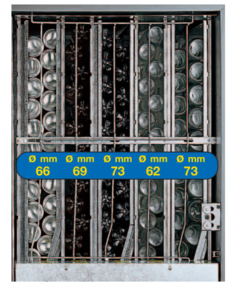
Die Einzelschächte können Produkte mit einem Durchmesser von 62 mm bis 73 mm ausgeben.
